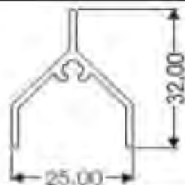
Louvre Y Section
