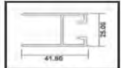
OXXO FIX STILE - FIXED SASH
