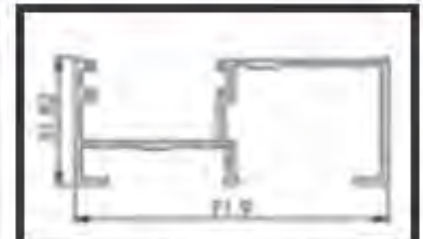
REVERSABLE JAMB - VISTA HEAD
